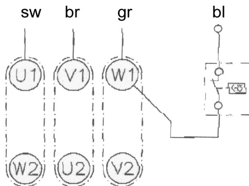
Motoranschluß Dreieck
